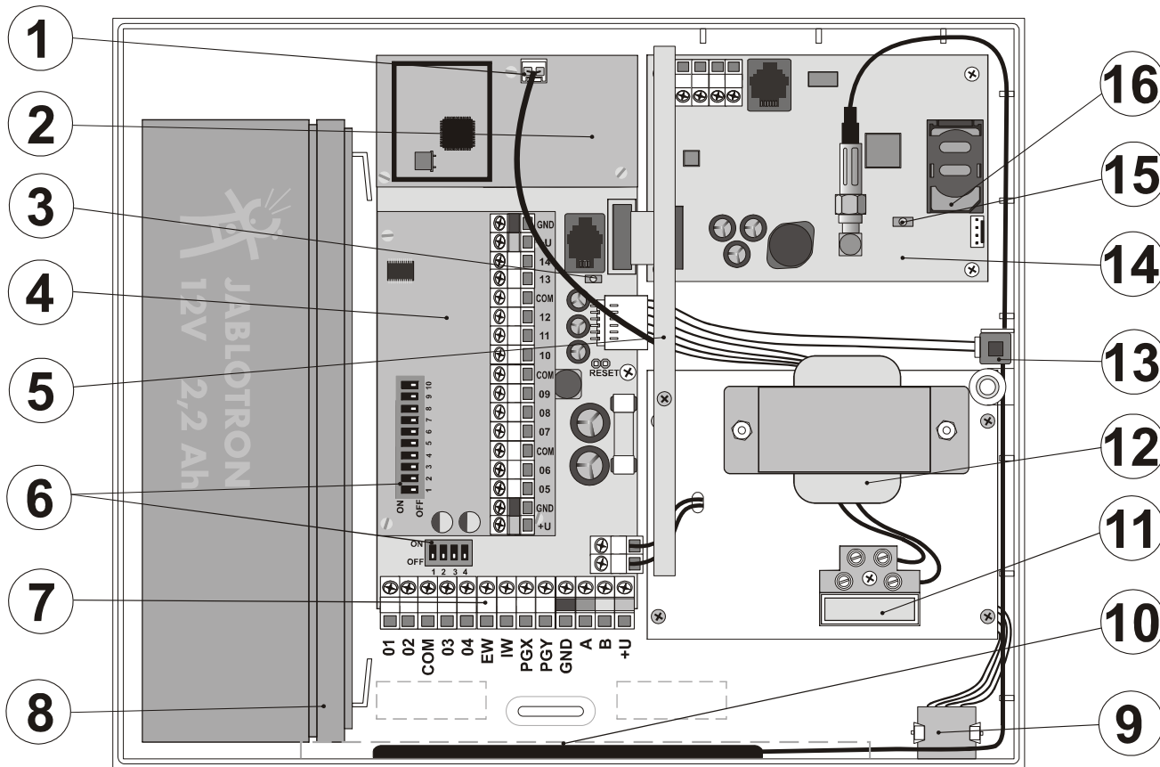
obr. 9 Rozmístění ve skříně ústředny
